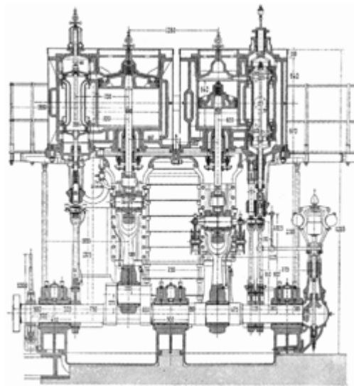
Fig. 17. Stående Verbundmaskin mit stähliger Kreuzkopfführung (stehtester Schnitt durch beide Zylinder).
